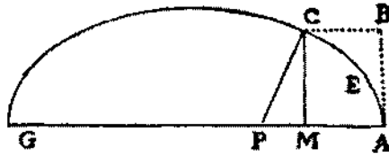
Figure 2: The case of the ellipse ( Géométrie , p. 343)
