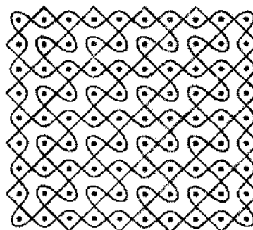
Dois sona construídos aplicando o mesmo algoritmo geométrico Figura 7
